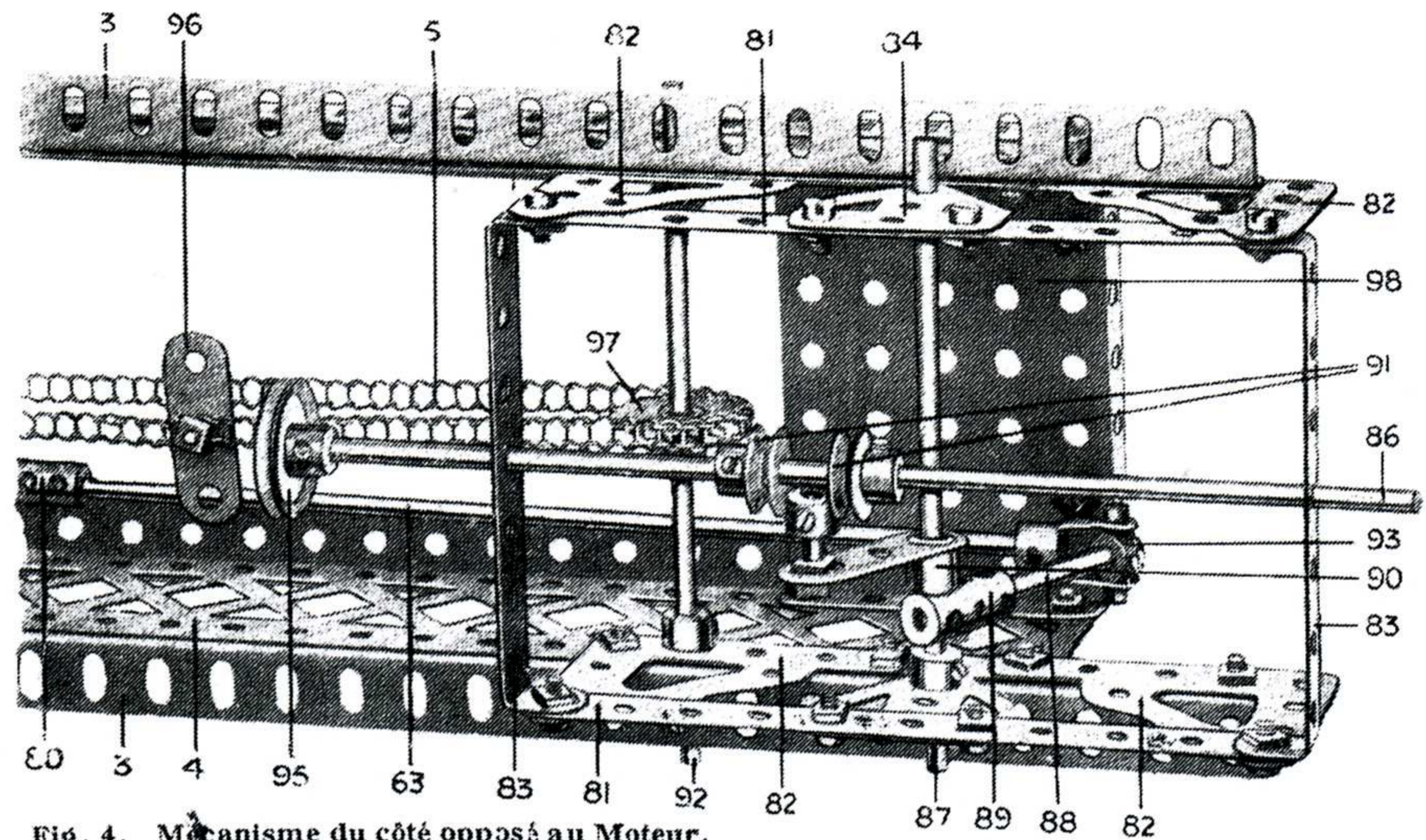
Fig. 4. Mécanisme du côté opposé au Moteur.
