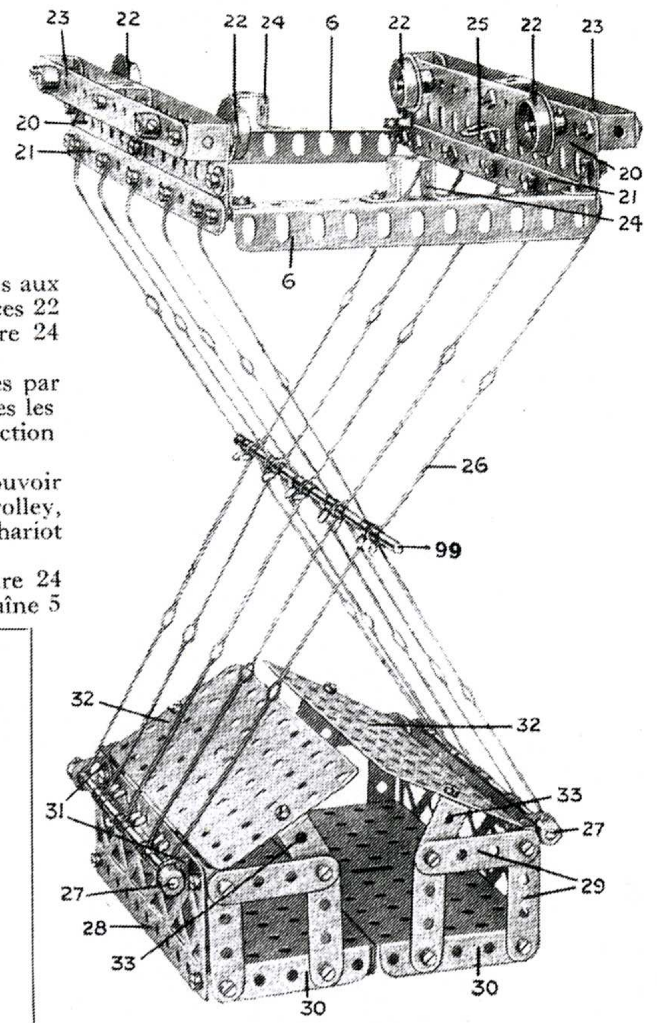
Fig. 5. Le trolley avec la nacelle suspendue.
